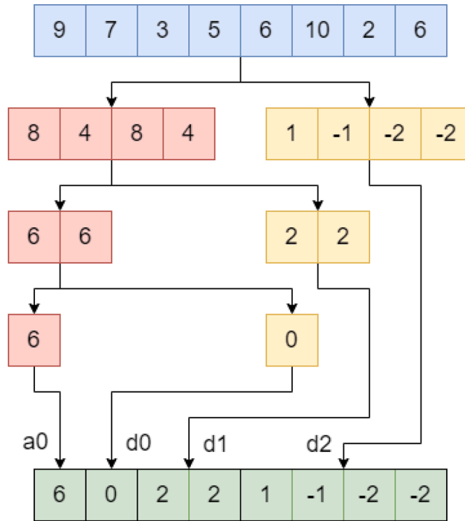
Fig. 4. Haar Transform/Decomposition.
