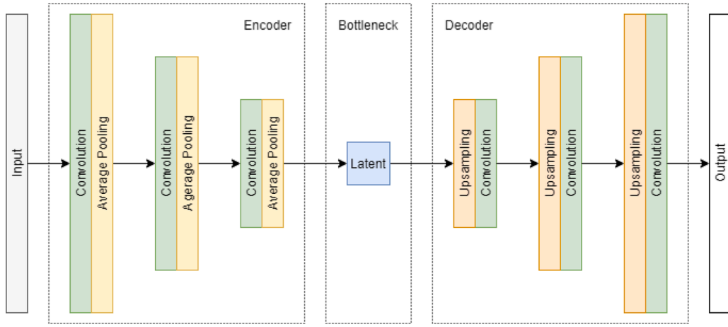
Fig. 17. Autoencoder architecture.
