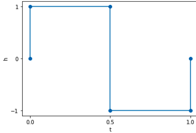
Fig. 3. Haar Wavelet.
